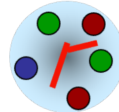
Pentaquark
