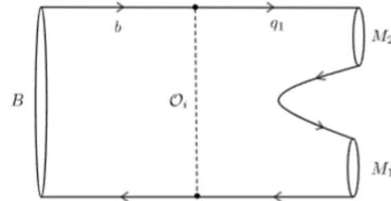
(d) CA: Connected Annihilation
