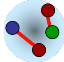
Tetraquark
